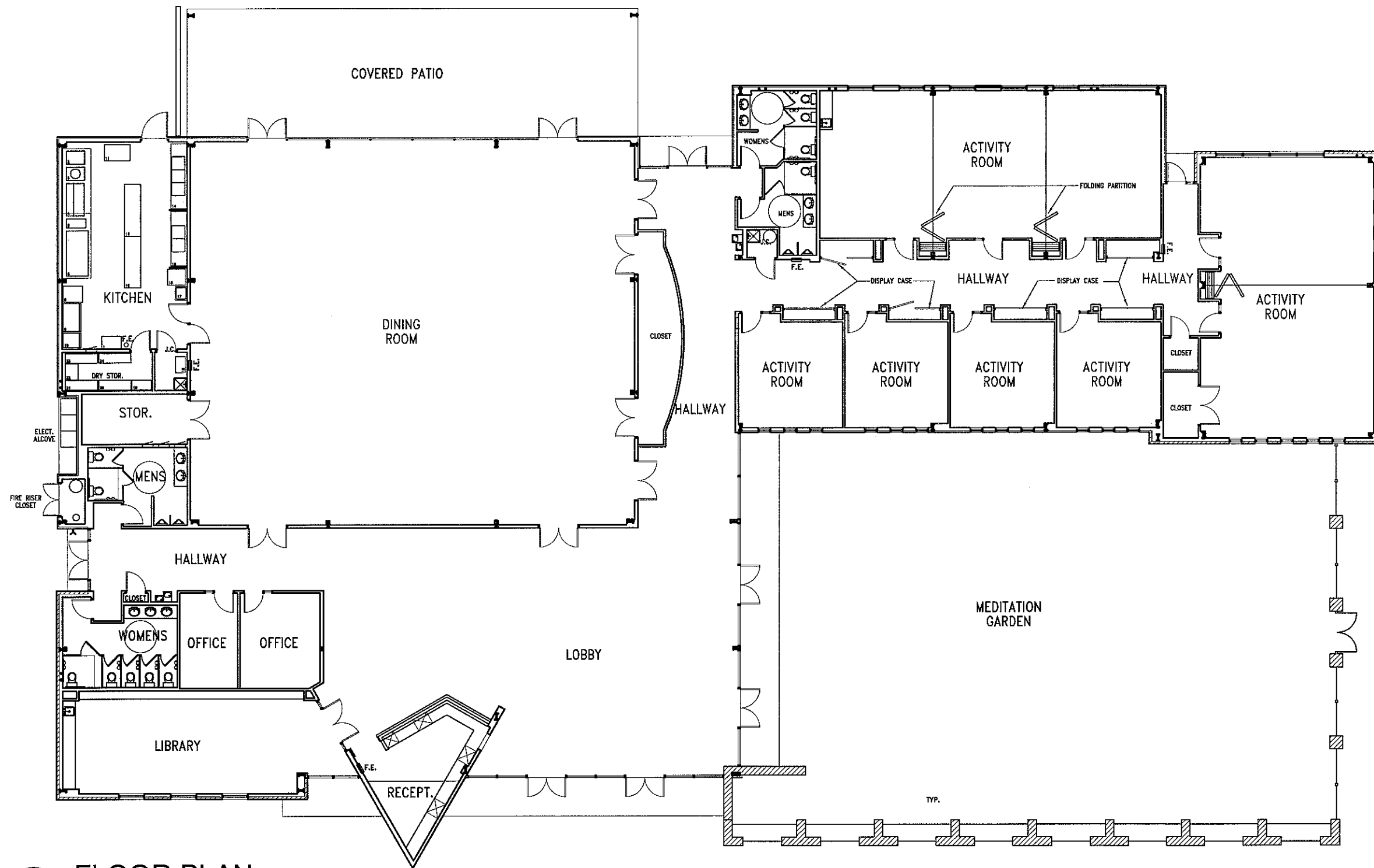
1 FLOOR PLAN N.T.S.
